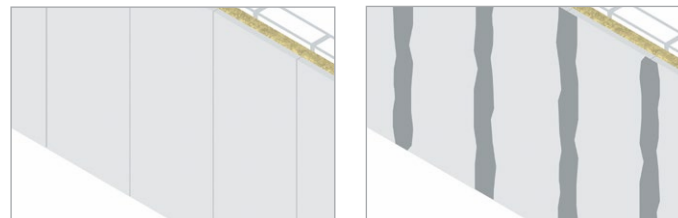
Рис. 14. Шпатлевание швов
