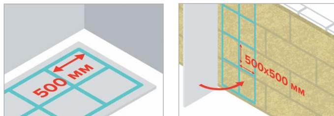
Нанесение на лист ГКЛ/ГВЛ
