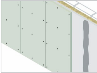
Рис. 16. Крепление листов ГКЛ/ГВЛ второго слоя
