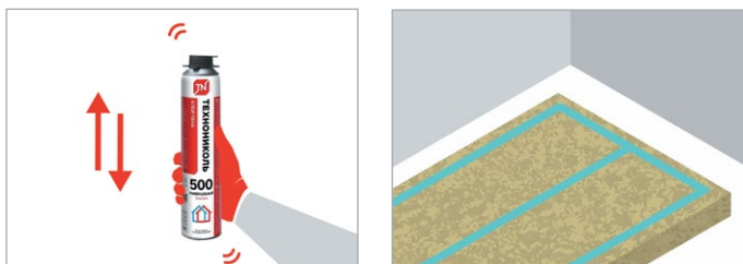
Рис. 6. Подготовка баллона и нанесение клея-пены
