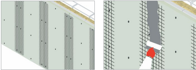
Рис. 17. Заделка швов
