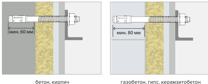
Рис. 20. Глубина установки анкера
