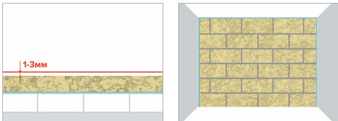
Рис. 10. Монтаж звукоизоляции
