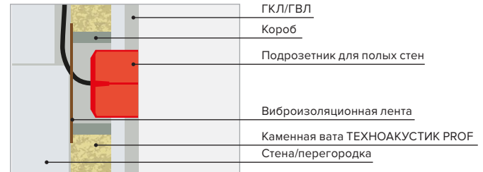
Рис. 18 в. Вариант монтажа электропроводки в несущей стене и подрозетника с монтажом в специальный короб
