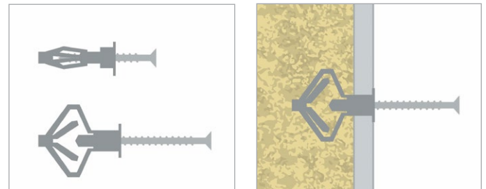
Рис. 19. Крепление элементов декора
